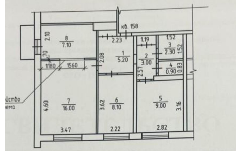
План квартиры после перепланировки
